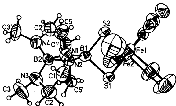
Fig. 3. ORTEP-Plot der Molekülstruktur von 6b . Thermische Ellipsoide mit 50% Wahrscheinlichkeit.
