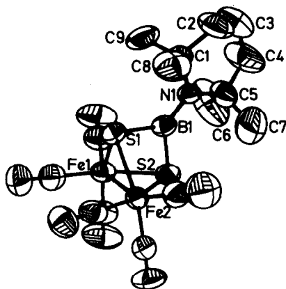
Fig. 1. ORTEP-Plot von \mu -(Tetramethylpiperidinoborandithiolato)bis(tricarbonylisen) (3). Thermische Ellipsoide mit 50% Wahrscheinlichkeit. H-Atome wurden der Übersichtlichkeit halber weggelassen.
