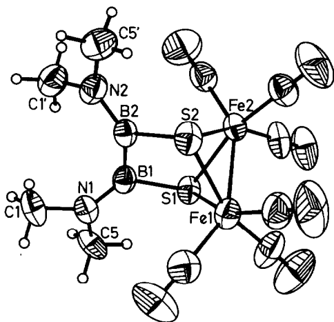
Fig. 2. ORTEP-Plot von \mu -Bis(dimethylamino)diboran(4)dithiolato)bis(tricarbonylisen) ( 4 ). Es wird nur eines der beiden kristallographisch unabhängigen Moleküle gezeigt.
